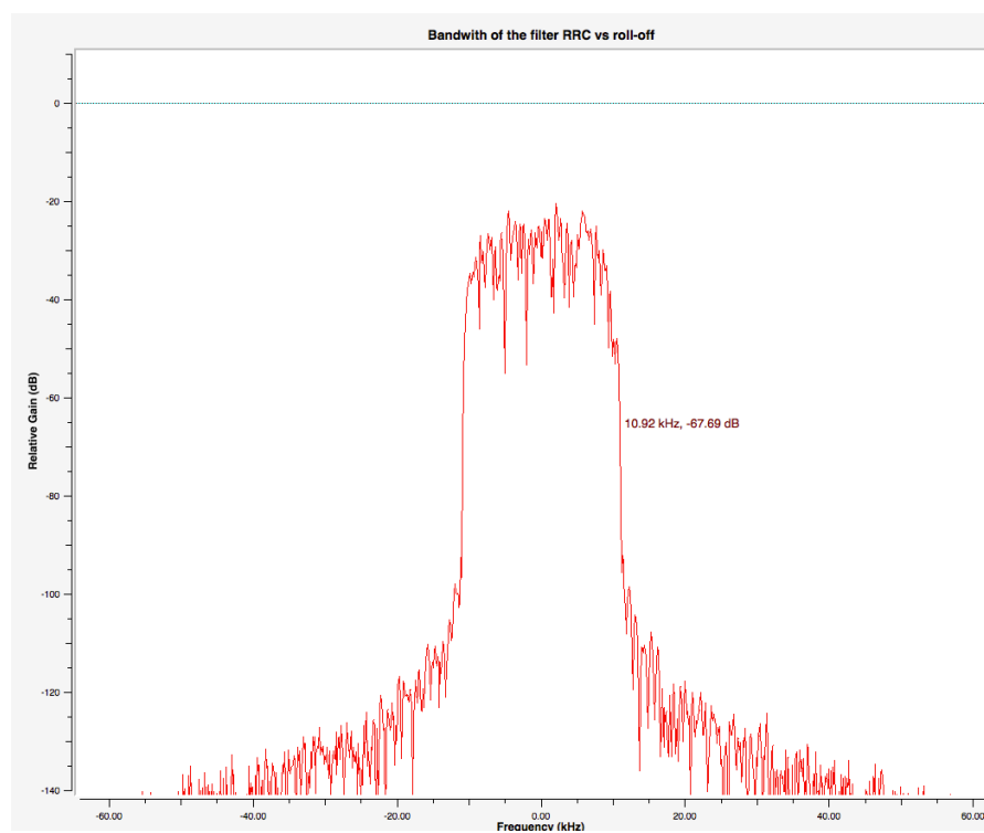
Figura 3. Densidad espectral de potencia de la secuencia de símbolos QPSK transmitida
